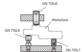
Anwendungsbeispiel verschiedener Pendelelemente mit O-Ring
